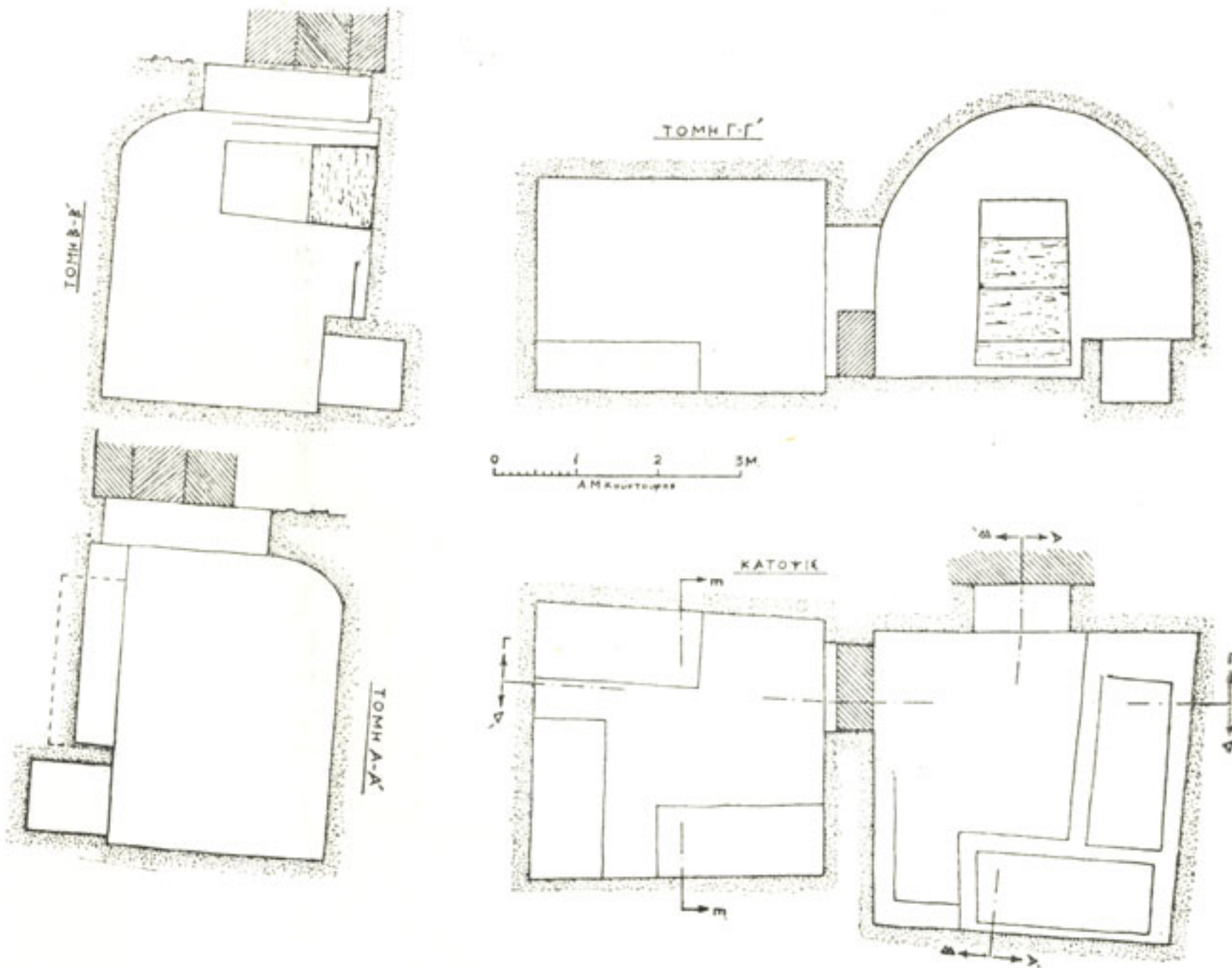
Είκ. 4. Βέροια. 'Υπόγειος λαξευτός τάφος μετά πλευρικού δωματίου έν τῷ συνοικισμῷ Καλλιθέας. Κάτοψις καί τομαί Α-Α', Β-Β' καί Γ-Γ'.
