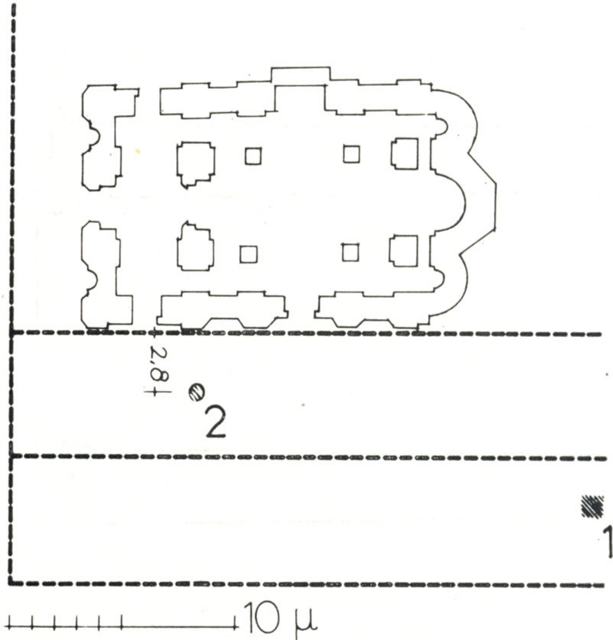
Σχ. 2. Ὁ αὐλόγυρος τῆς Παναγίας τῶν Χαλκέων καὶ ἡ θέση τῆς ὑπόγειας στοᾶς. 1) Τμῆμα κτιστῆς καμάρας. 2) Στόμιο πηγαδιοῦ.
