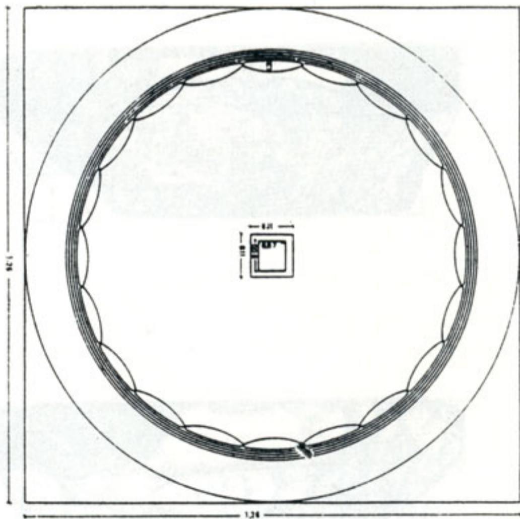
Σχέδιο 2. Το μεγάλο κιονόκρανο αρ. 1 (αποκατάσταση).
