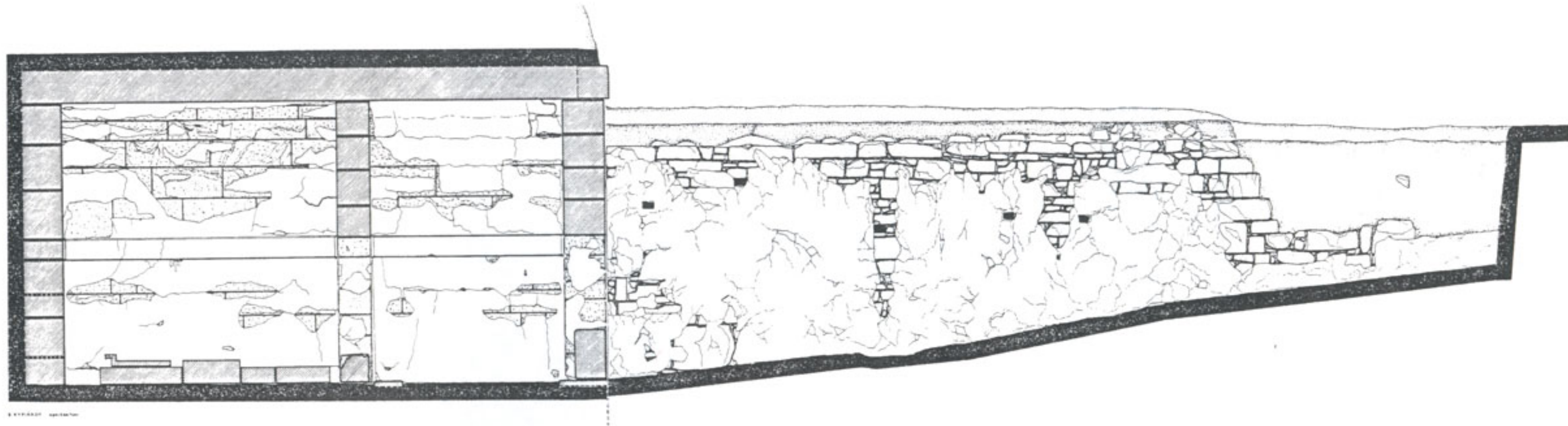
Σχ. 2. Τομή κατά μήκος (ανατολική) του μακεδονικού τάφου ΣΤ' με τις σαρκοφάγους της Πέλλας.
