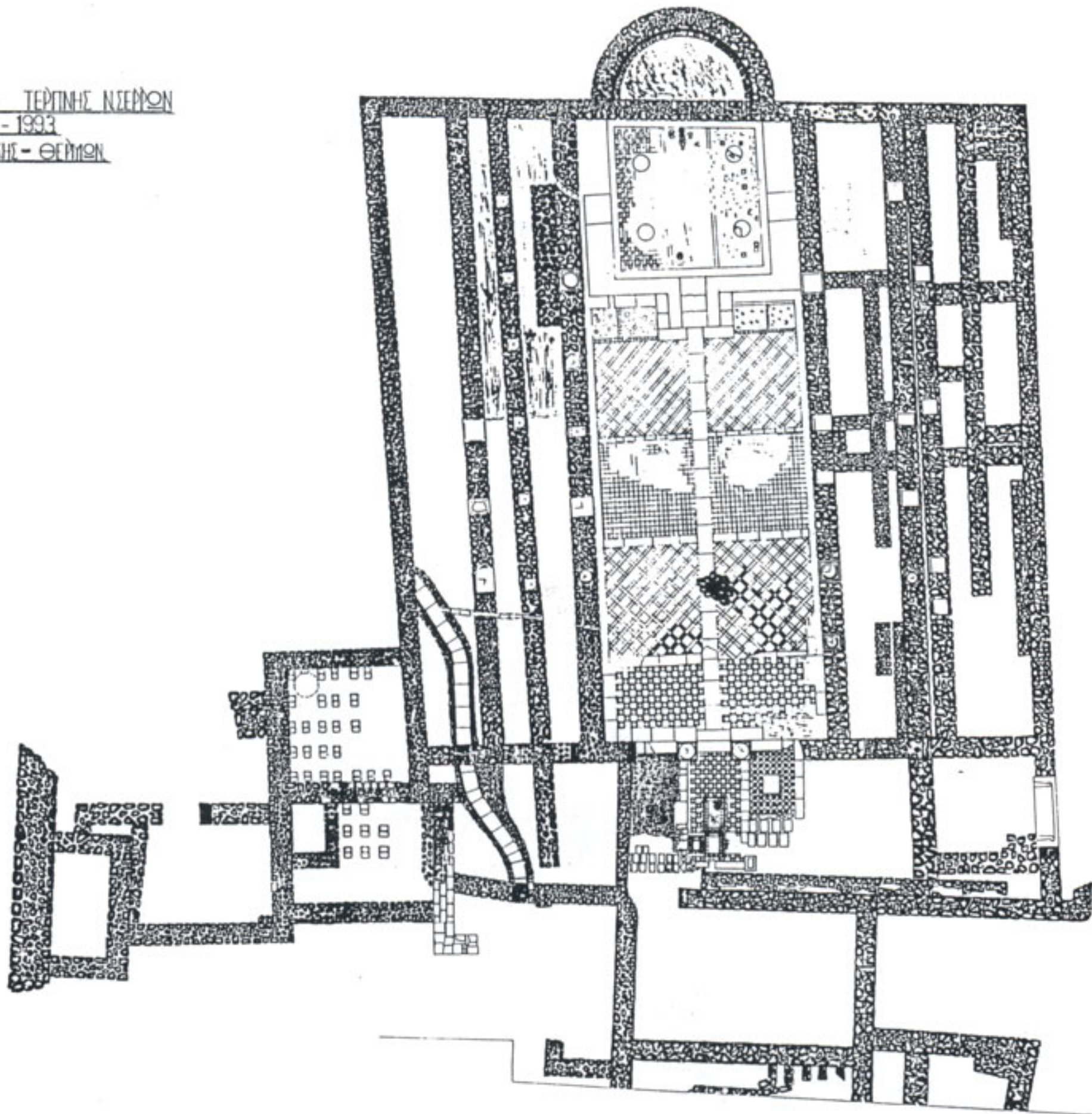
Σχ. 3. Κάτοψη βασιλικής-θερμών.
